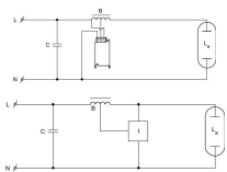
Caractéristiques Philips HID-HighPower BSN 1000 L78 230/240V 50Hz HP-257
